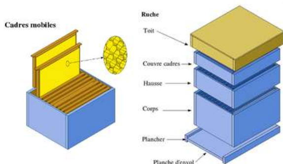
Corps de ruche à cadres mobiles
